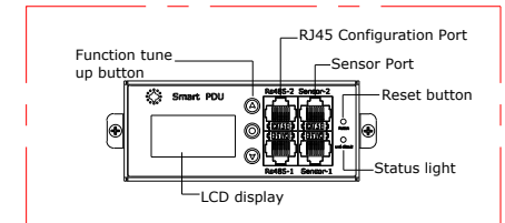
DETAIL A 2 : 1
